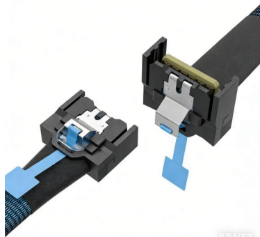
MCIO 4X 直头对4X 弯头 PCIe Gen5 高速数据线
