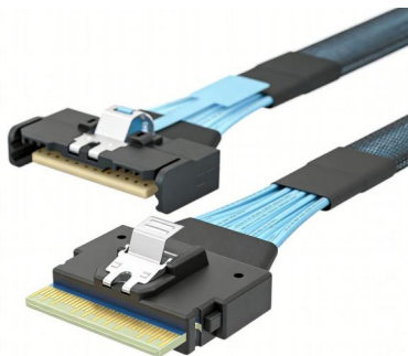
MCIO 8X 转SLIMSAS SFF-8654 8X Gen4 slimSAS 高速线
